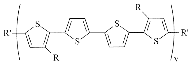
(A4)
