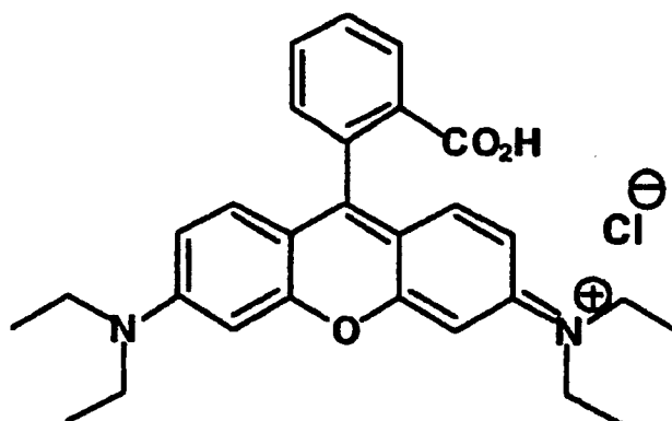
Rhodamine B
