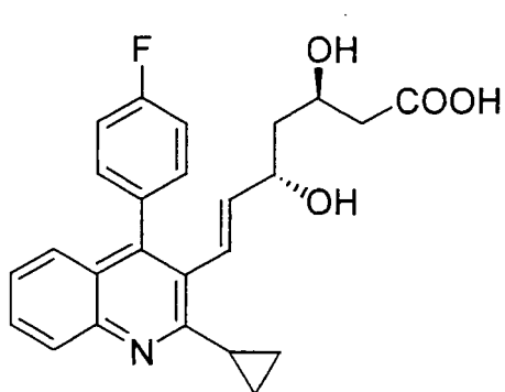
Pitavastatin
