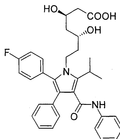
Atorvastatin
