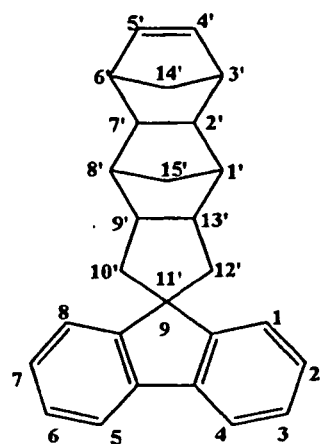
(15) Spiro [fluorene-9,11'-pentacyclo [ 6.5.1.1 3,6 .0 2,7 .0 9,13 ] [4] pentadecene]
