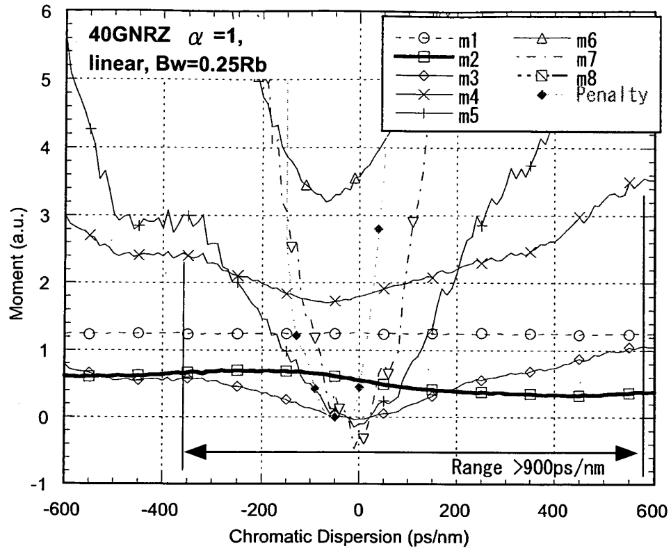
Fig.12 A NRZ
