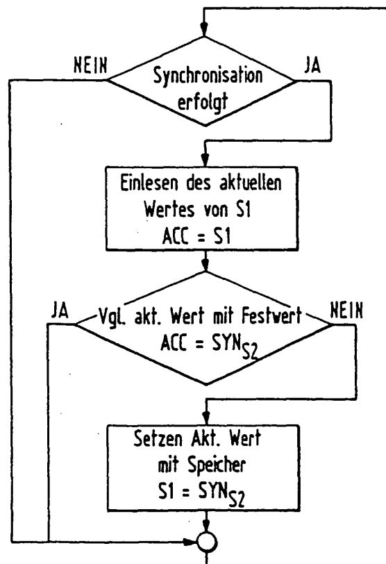
Ablaufdiagramm Synchronisation
