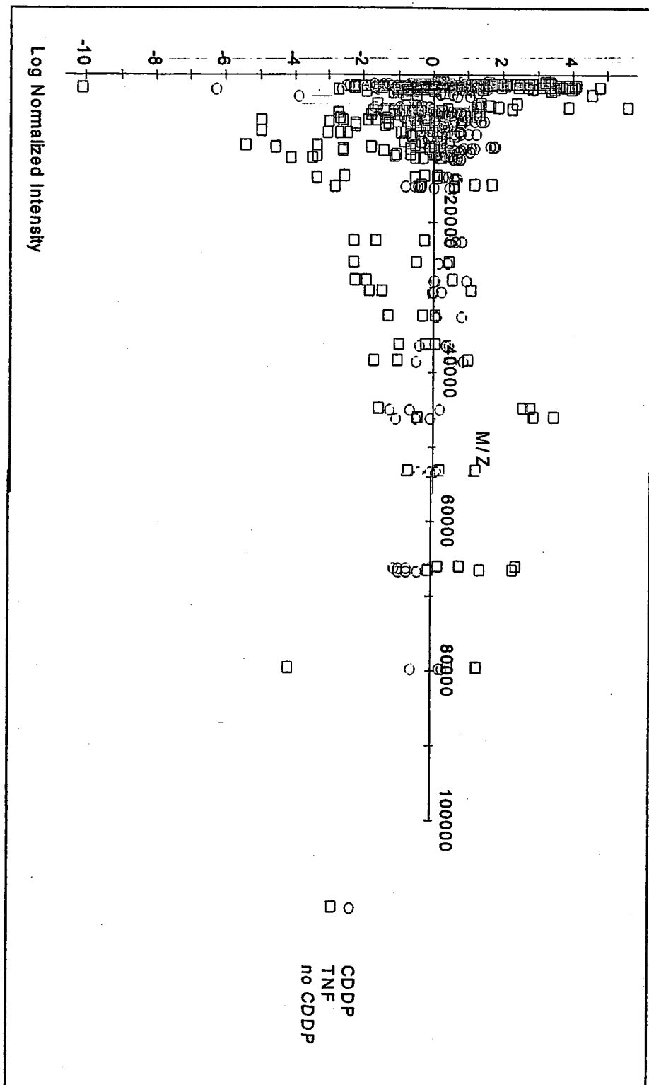
Figure 13 : représentation des différences entre les spectres des 3 phénotypes sans TNF ni CDDP, avec TNF et avec CDDP
