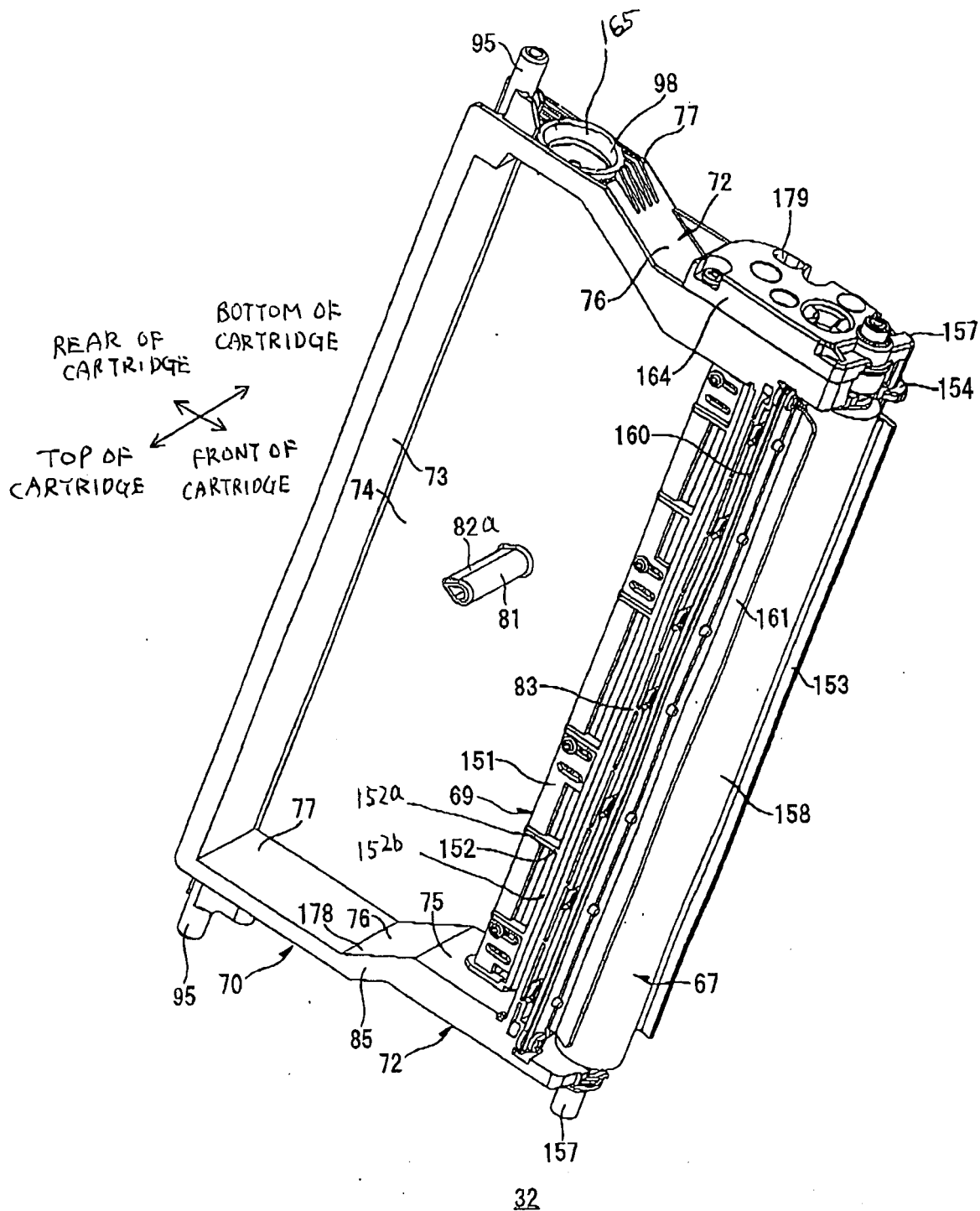
FIG. 15(b)
