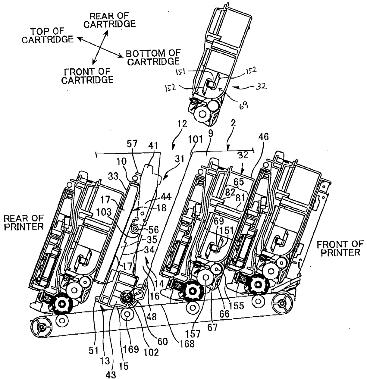
FIG.18
