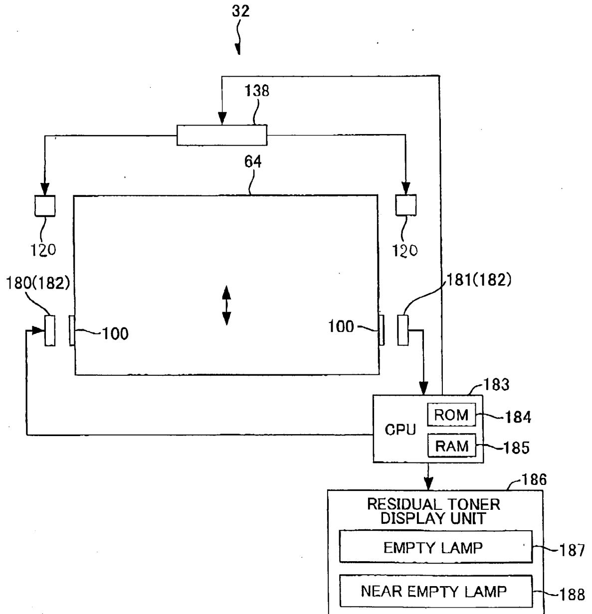
FIG.27
