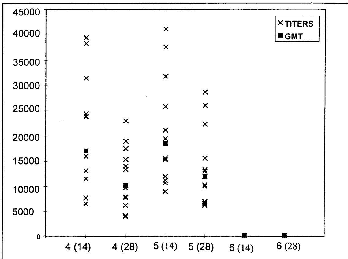
Figure 5, Anti HSV gD titres (see example 3).
