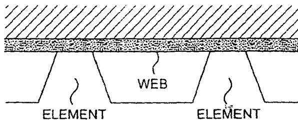
FIG. 17A
