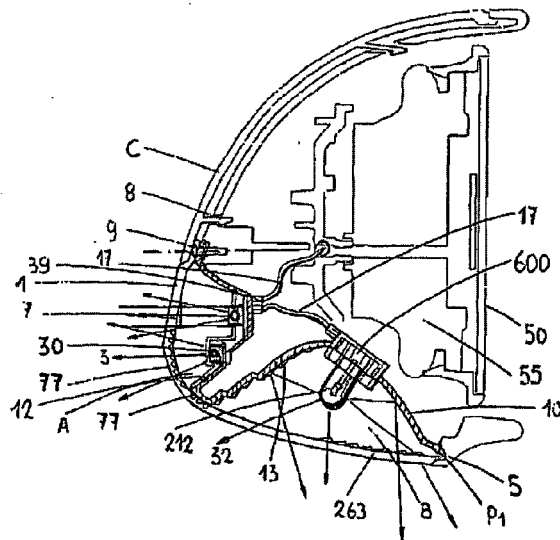
FIG.115 SECTION A-A
