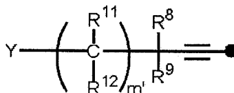
[Chem. 3]
