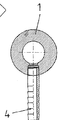
[ - ]_n
