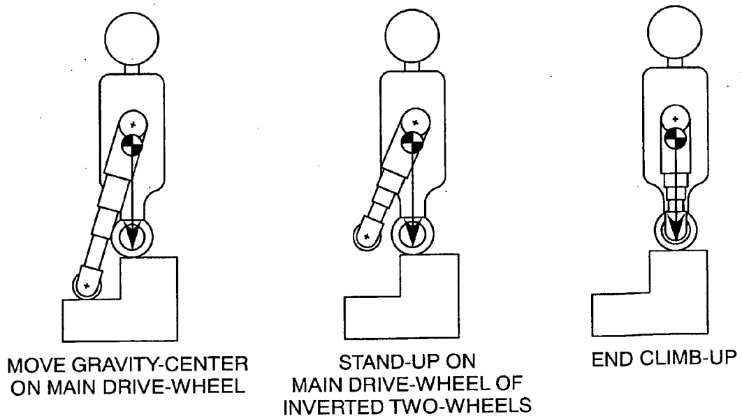
FIG.14(e) FIG.14(f) FIG.14(g)
