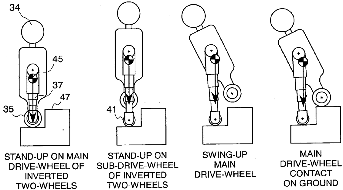
FIG.14(a) FIG.14(b) FIG.14(c) FIG.14(d)
