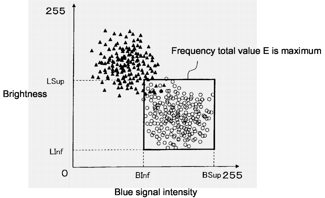
FIG. 17B
