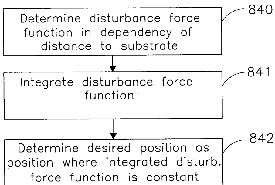
Fig. 8E
