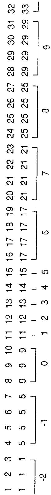
Fig.17 (d) quantization
