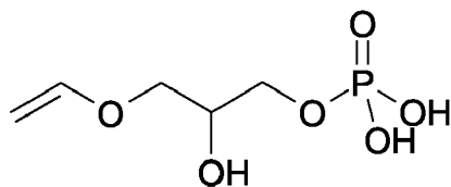
Phosphorsäuremono-(1-phosphonoxymethyl-2-vinyloxy-ethyl)-ester
