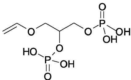
Phosphorsäuremono-(3-allyloxy-2-hydroxy-propyl)ester
