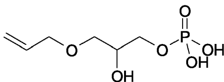
Phosphorsäure mono-2-(allyloxy-1-phosphonoxymethyl-ethyl)ester
