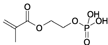
Phosphorsäuremono-(-2-hydroxy-3-vinyloxy-propyl)ester
