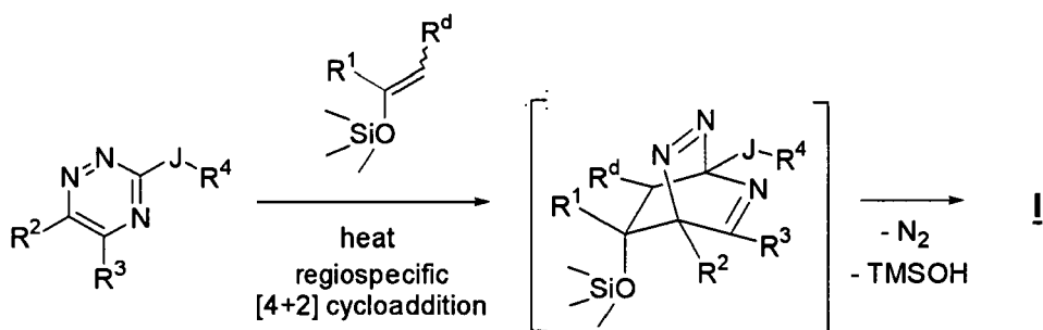
Scheme 1.e
