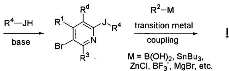
Scheme 1.e
