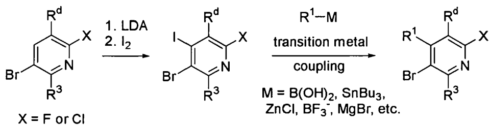
Scheme 1.d
