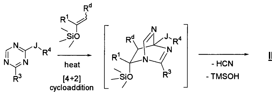
Scheme 2.e
