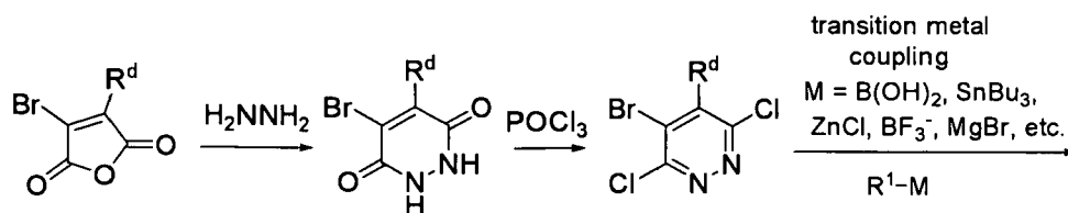
Scheme 3.b
