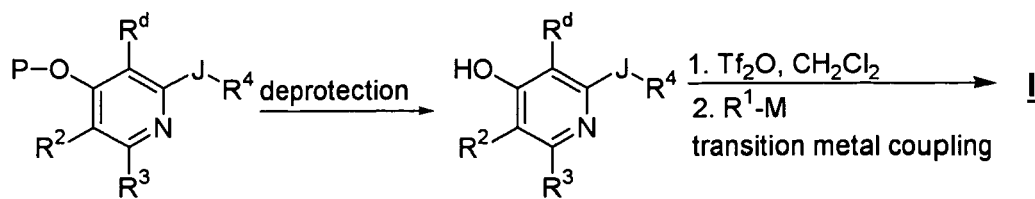
Scheme 1.d
