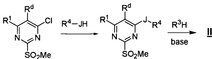
Scheme 2.e
