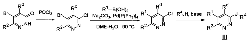
Scheme 3.a
