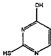
2-Thiouracil
