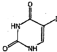
5-Iodouracil
