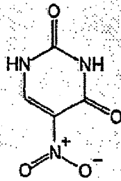
5-Nitrouracil
