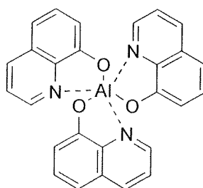
Alq
