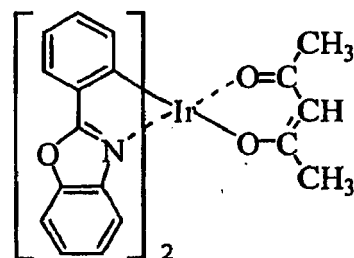
(K-14)
