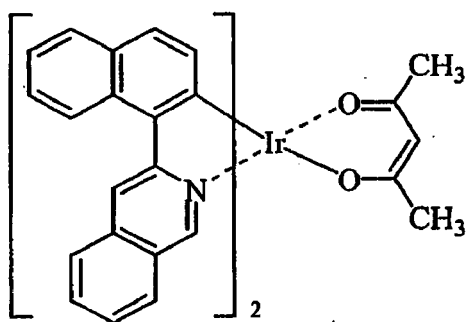
(K-19)
