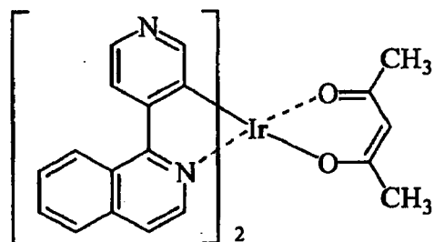
(K-20)
