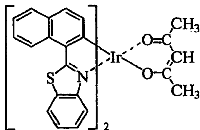
(K-16)
