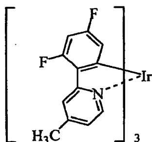
(K-9)
