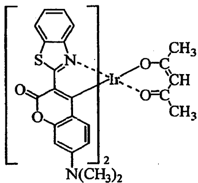
(K-19)
