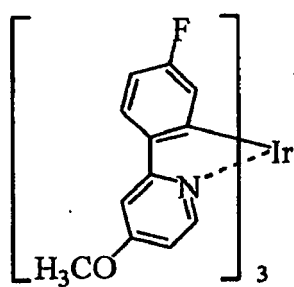
(K-4)
