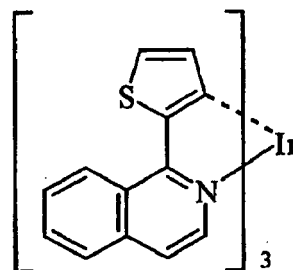
(K-22)
