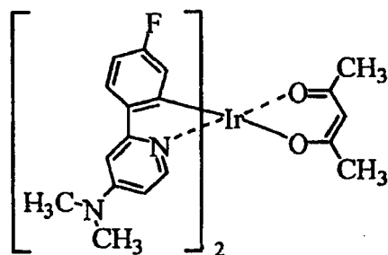
(K-8)
