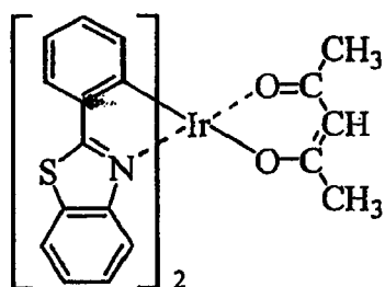
(K-15)
