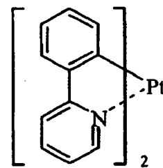
(K-14)
