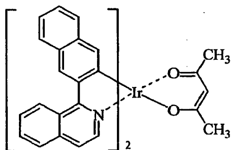
(K-18)
