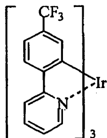
(K-12)
