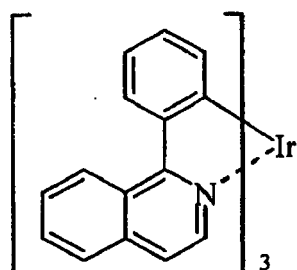
(K-21)
