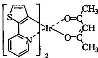
(K-13)
