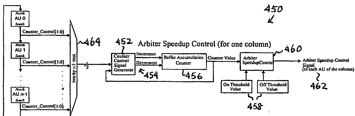
Output Port (column) Arbitrer Speedup Control
