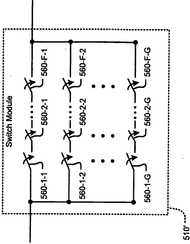
FIG. 19B
