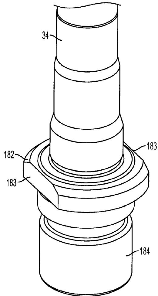
FIG. 32
