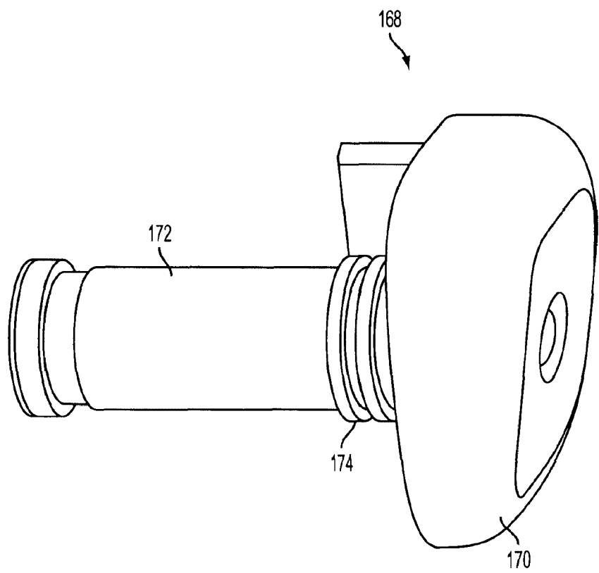
FIG. 31
