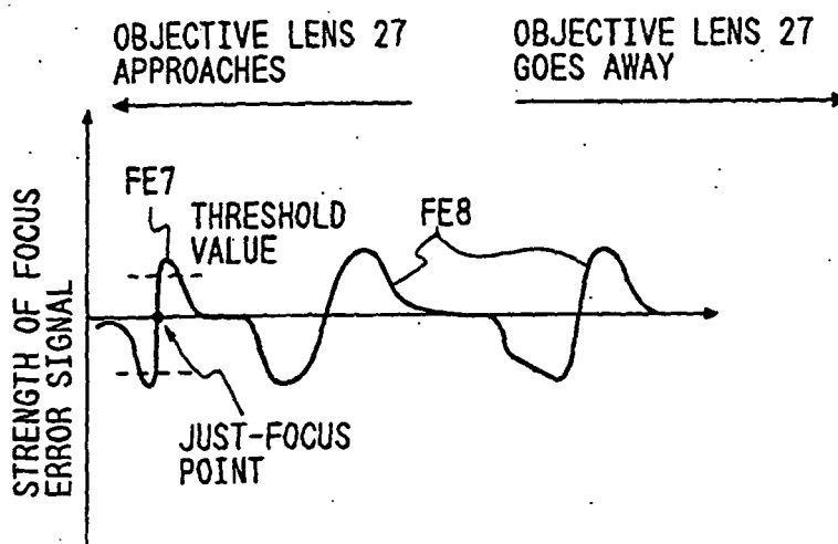
FIG. 36B
