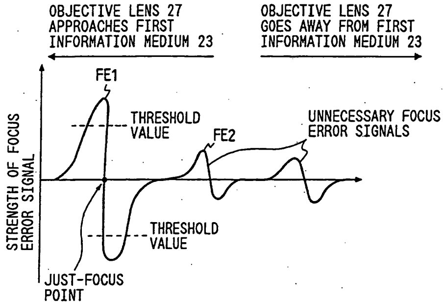
FIG. 35A
