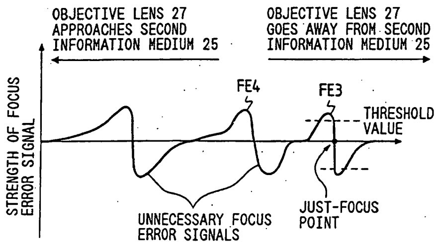
FIG. 35B
