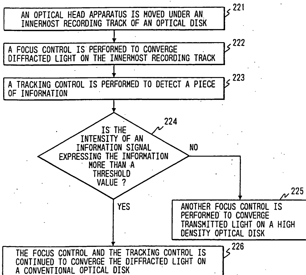
FIG. 58
