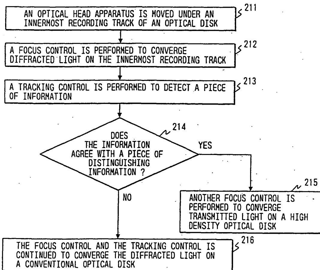
FIG. 56
