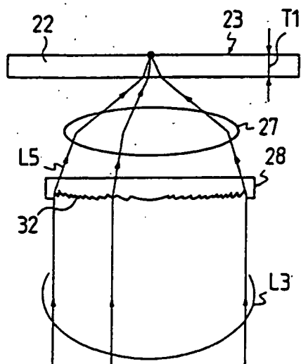
FIG. 15B
