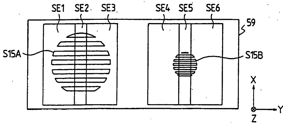
FIG. 42C
