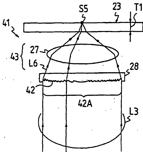
FIG. 16A
