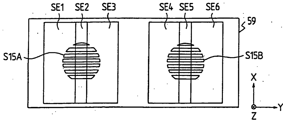
FIG. 42B
