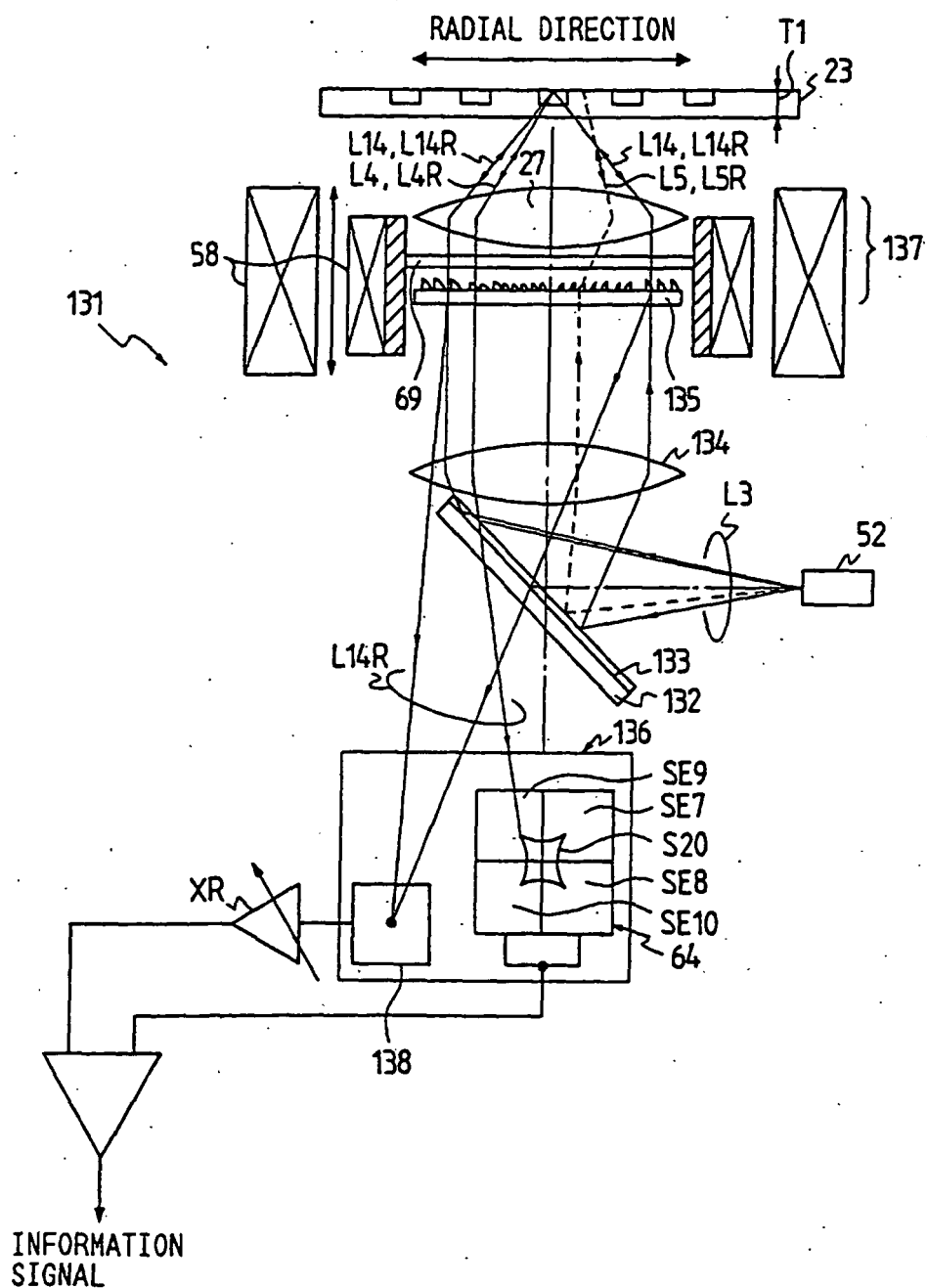
FIG. 45
