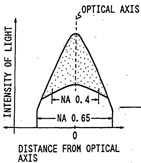
FIG. 18A
