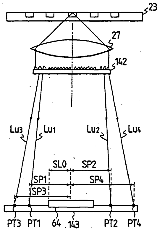
FIG. 49A
