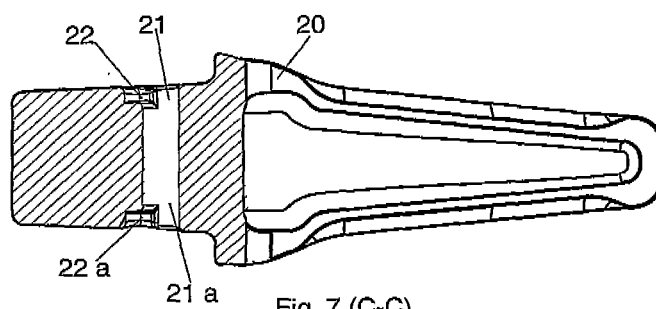
Fig. 7 (C-C)
