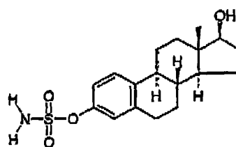
17β oestradiol-3-sulphamate
