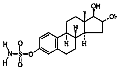
oestriol-3-sulphamate
