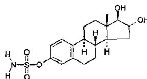
oestriol-3-sulphamate
