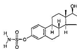
17β oestradiol-3-sulphamate
