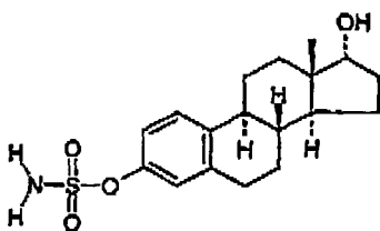
17α oestradiol-3-sulphamate
