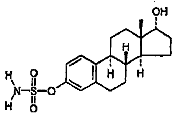
17α oestradiol-3-sulphamate
