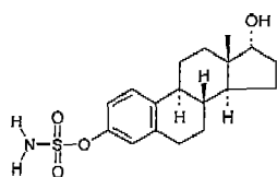
17α oestradiol-3-sulphamate
