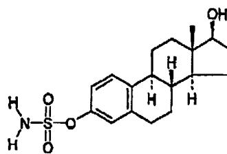
17β oestradiol-3-sulphamate
