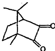
Camphorquinone
