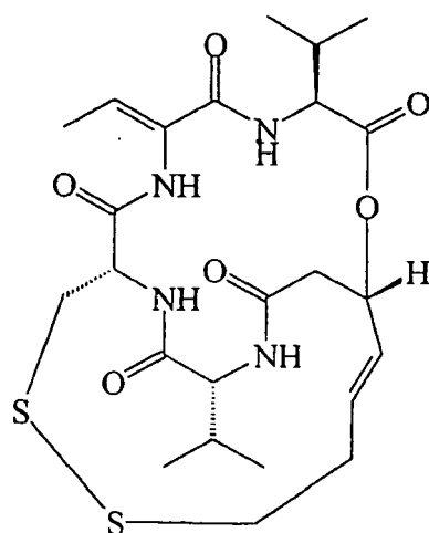
FR901228
