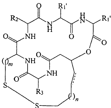
(IV)
