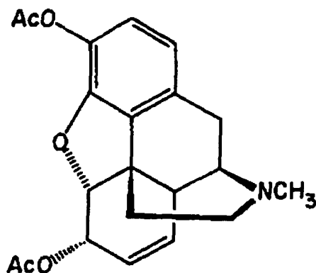
HEROIN
