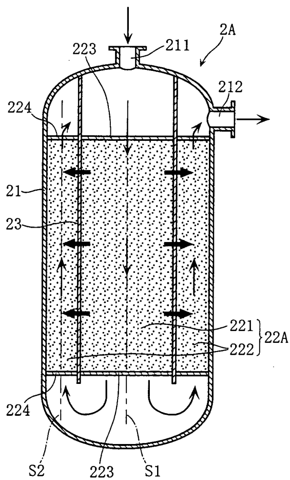
FIG. 4B
