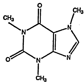
CAFFEINE
