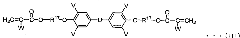
[Chem 5]
