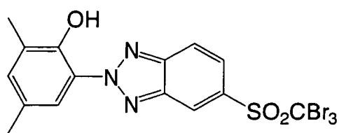
H-22
