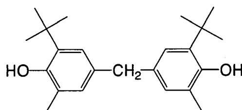
(R' - 26)
