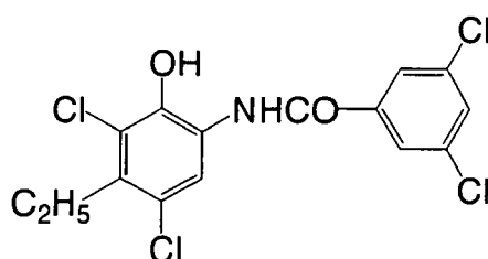
(A' '-12)
