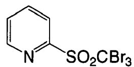
H-3
