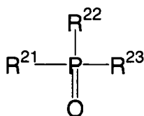
General Formula (D)
