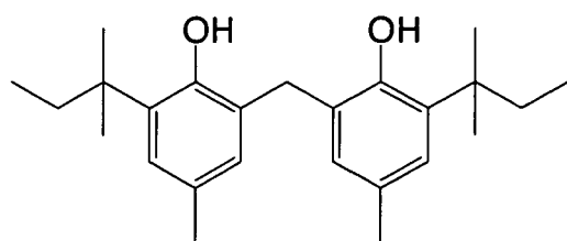
(R-13)
