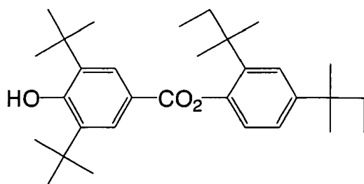
(R' - 23)
