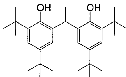
(R' - 11)
