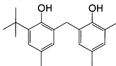
(R-14)
