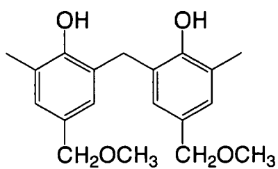
(R' ' - 1 7 )
