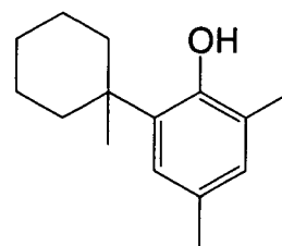
(R' - 22)
