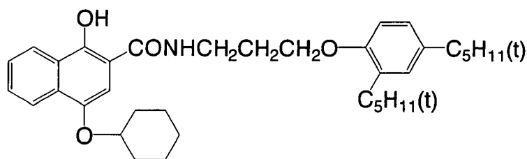
(A' '-9)
