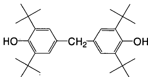
(R - 31)
