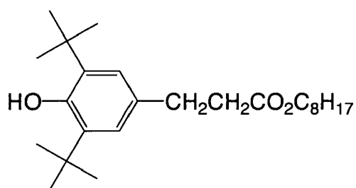
(R' - 29)
