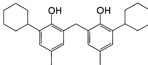
(R' ' - 1 2 )
