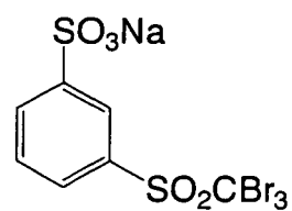
H-23
