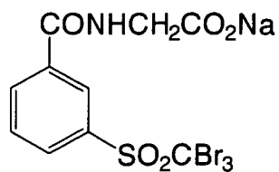
H-14
