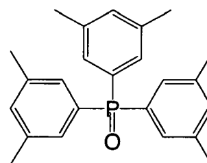
(D-6)
