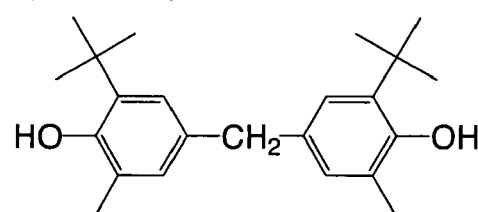
(R - 32)
