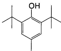
(R' - 21)
