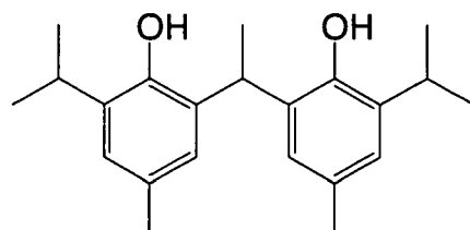
(R-12)
