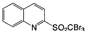
(H-4)
