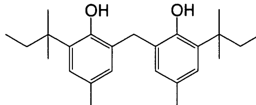
(R' - 10)
