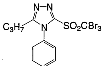
(H - 10)
