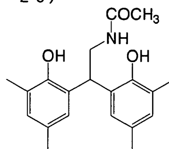
(R' - 20)
