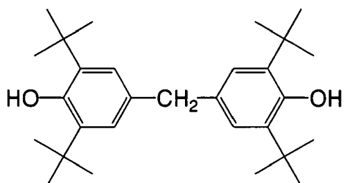
(R' - 25)
