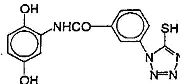
I'' - 3)
