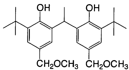
(R' - 23)
