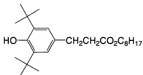
(R' - 24)
