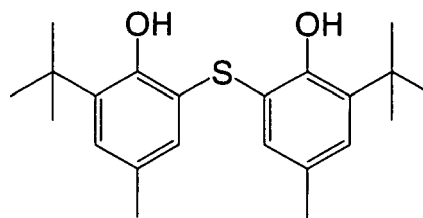
(R' - 20)
