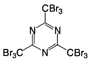
H-7
