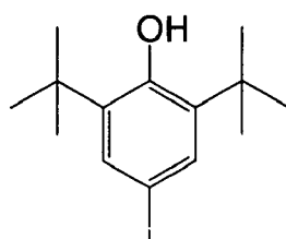
(R' - 21)
