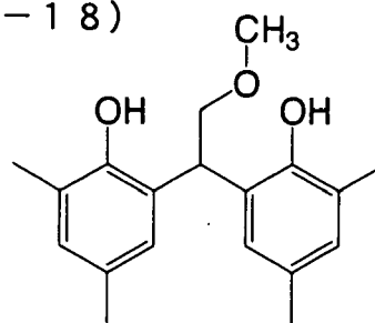
(R' - 20)
