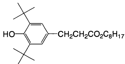
(R' - 24)
