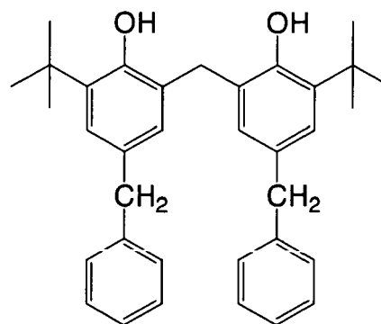
(R' - 22)
