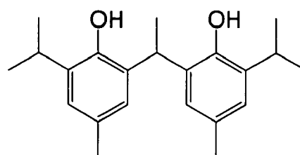
(R' - 10)
