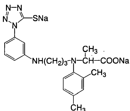
(I - 1)
