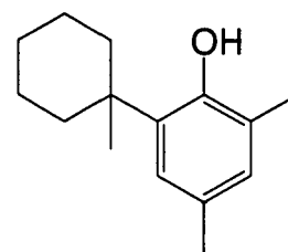
(R' - 26)
