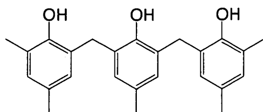
(R' - 25)
