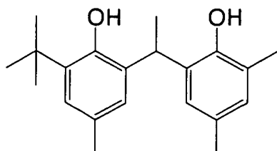
(R' - 15)
