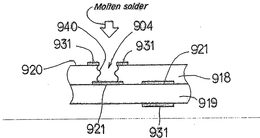
FIG. 49
