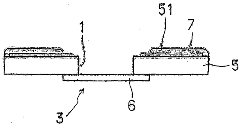
FIG. 58
