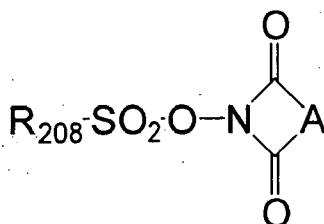
ZV
