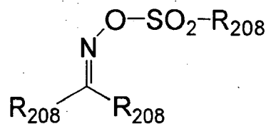
ZVI
