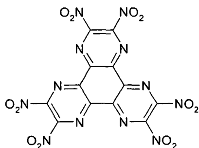
Formula Ic
