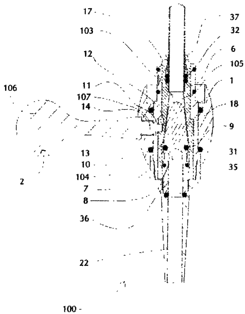
Fig. 4 Section B-B
