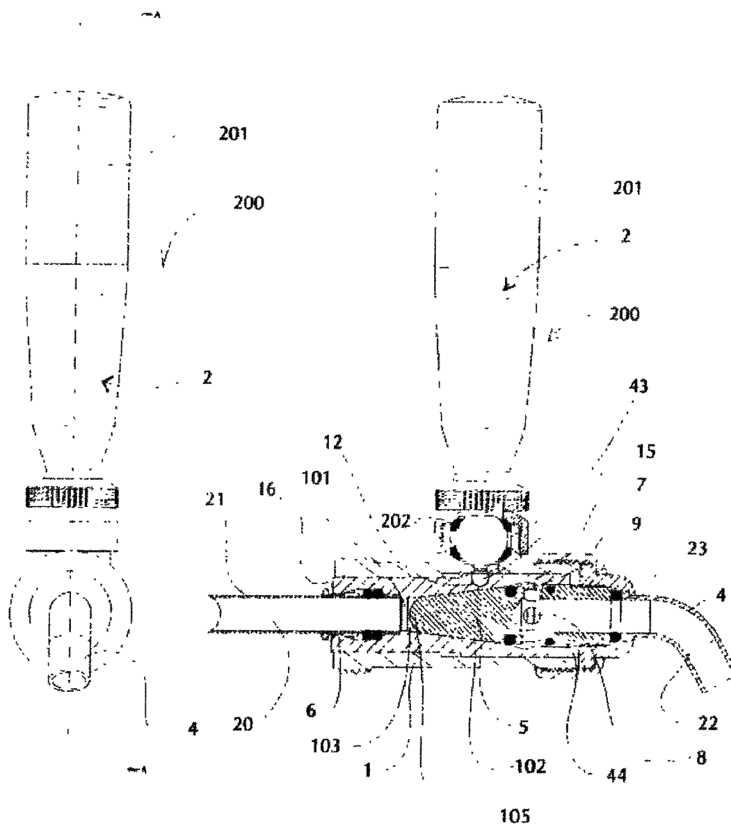
Fig. 9 Section A-A
