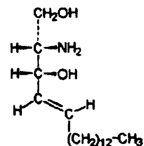
(Sphingosin)
