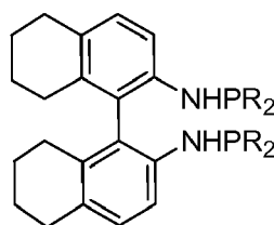
BINAPAN R = aryl, alkyl
