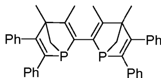
BIPNOR
