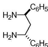
Dppn
