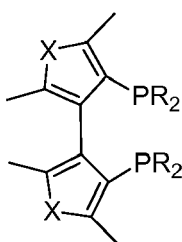
TMBTP R = aryl, alkyl X = O, S, N
