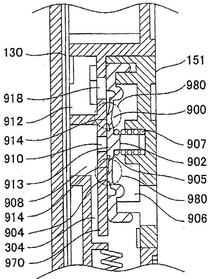
FIG. 19B
