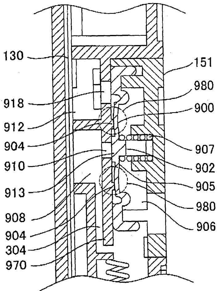
FIG. 15B
