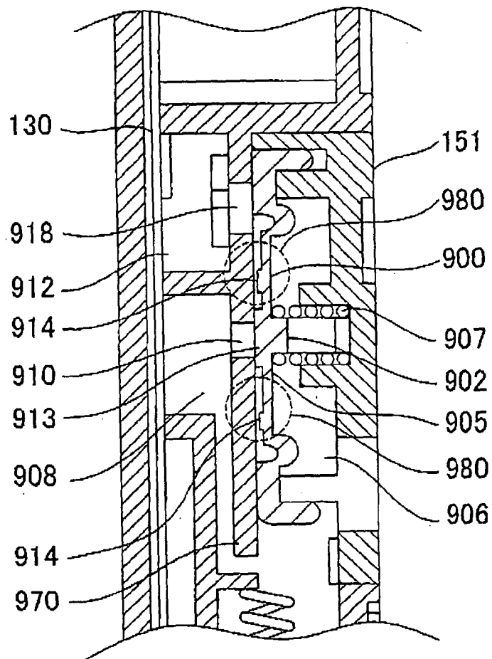
FIG. 17B
