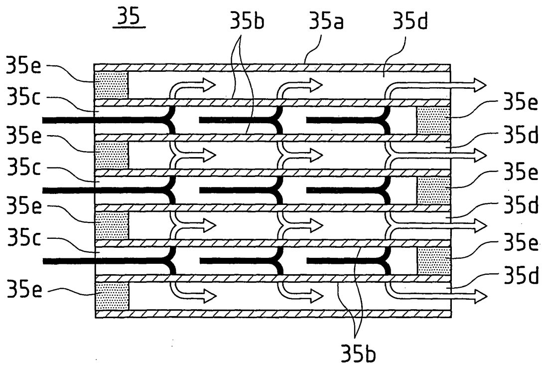
FIG.33
