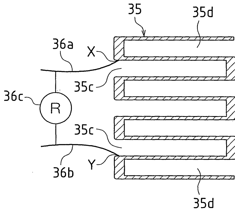
FIG.35
