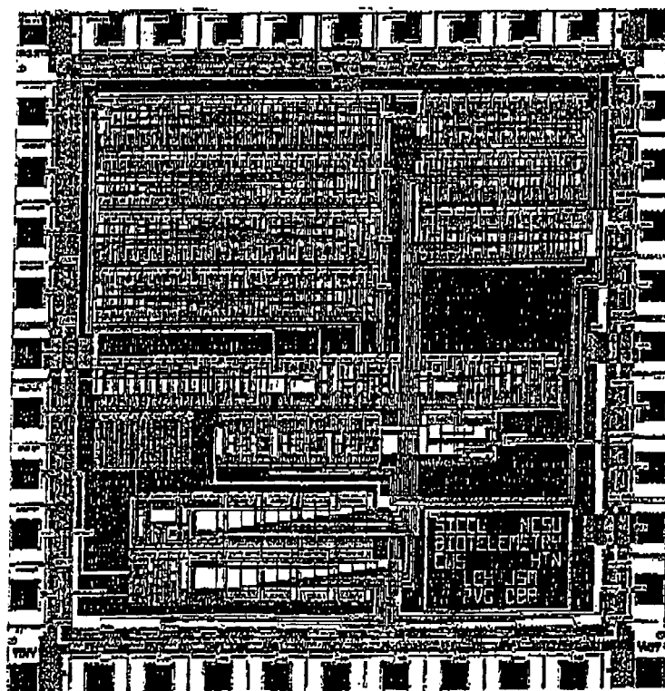
IC LAYOUT
