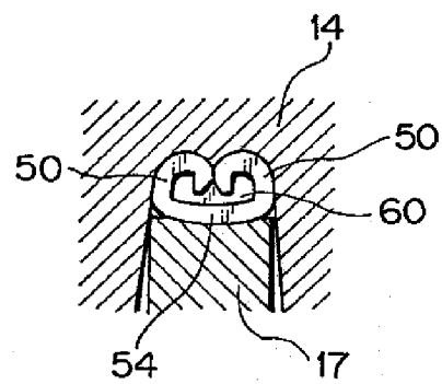
FIG. 6D
