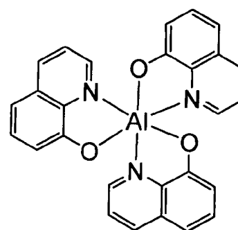
Alq
