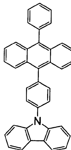
CzPA
