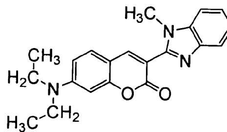
Coumarin30
