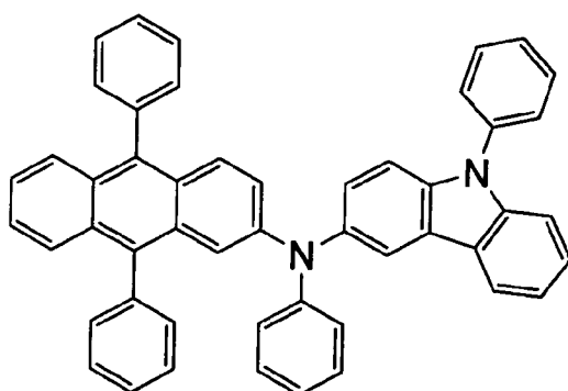
2PCAPA
