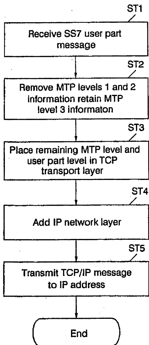
FIG. 19
