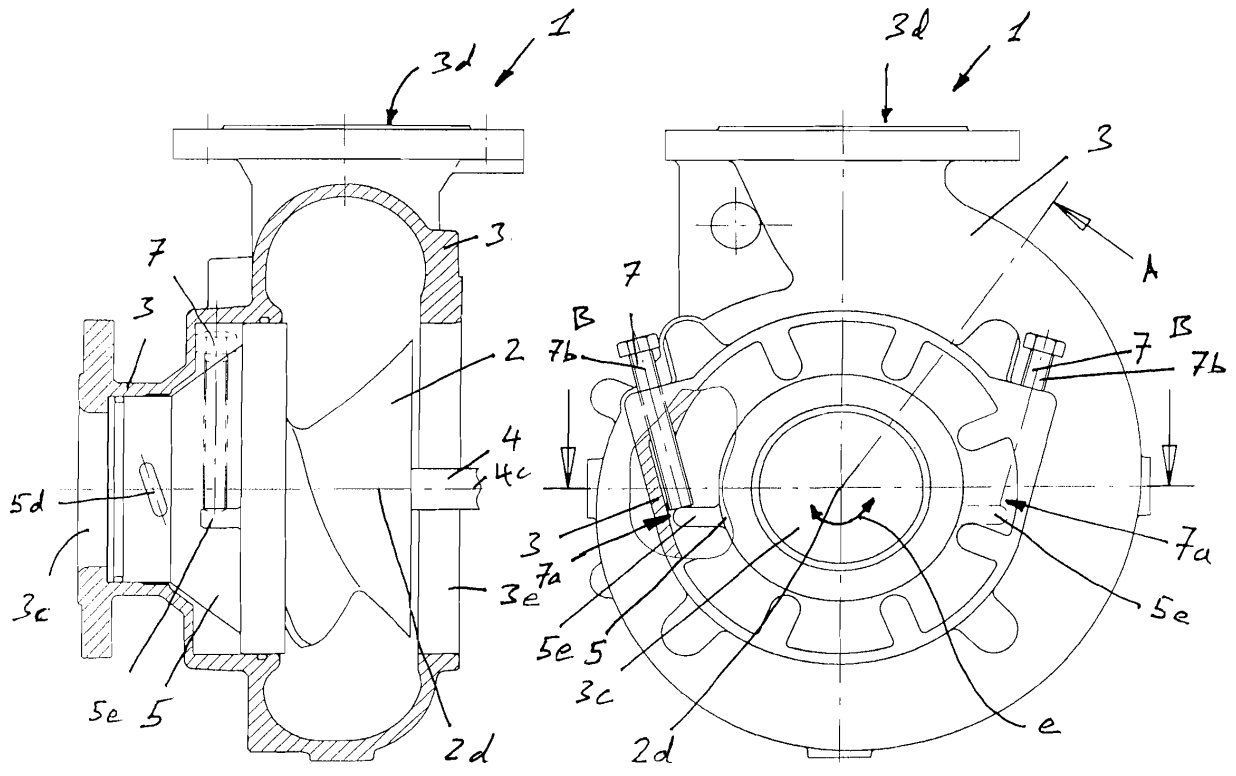
Fig. 3(A-A)
