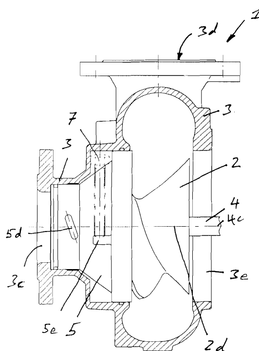
Fig. 3(A - A)
