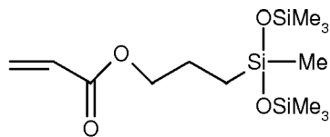
acryloxypropylbis(trimethylsiloxy)méthylsilane
