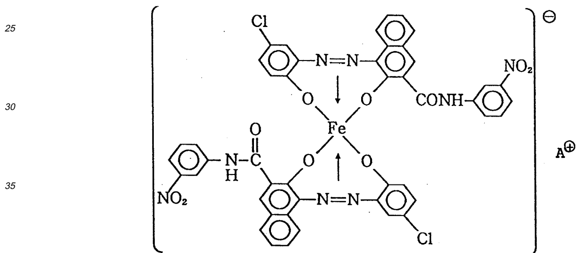
Azo ion complex (3)
